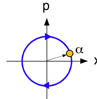
Phasenraum-Darstellung
